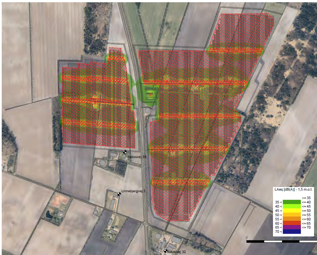
Figur 6-2 Støjudbredelseskort ved nærmeste boliger om natten.
