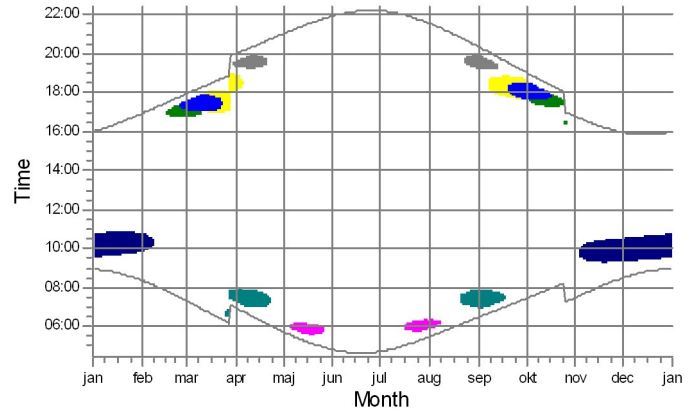
2: Siemens Gamesa SG 6.0-155 6000 155.0 !O! hub: 90,0 m (TOT: 167,5 m
