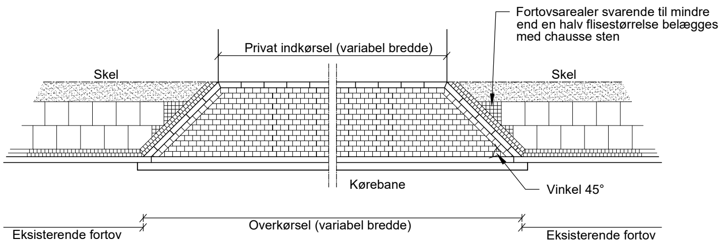
Mål: 1:100
